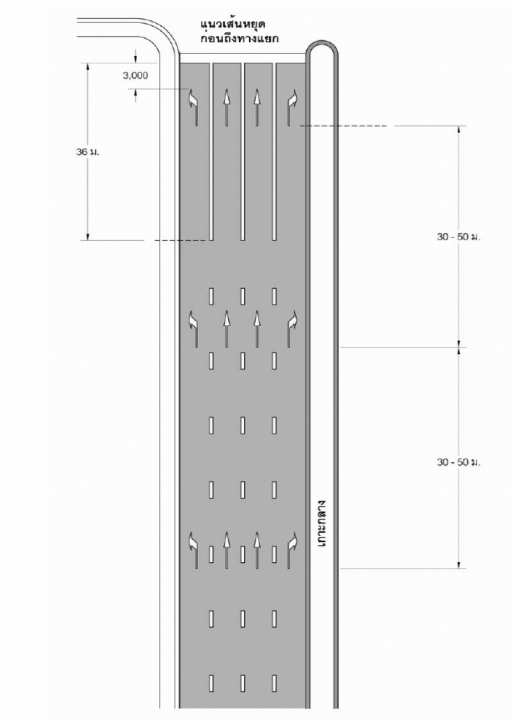
มาตรฐานตำแหน่งลูกศรบนช่องจราจรก่อนถึงทางแยก
