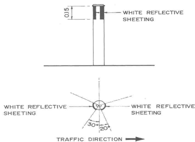
รูปที่ 7-2 การคิดแผ่นสะท้อนแสงในระบบราวกันอันตรายแบบเคเบิล
